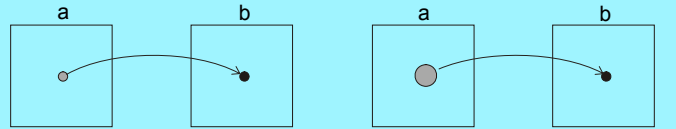
bodové operace
