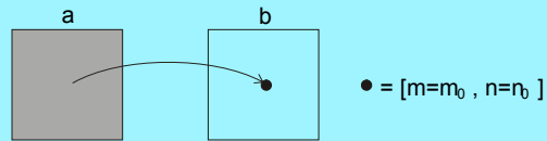
globální operace
